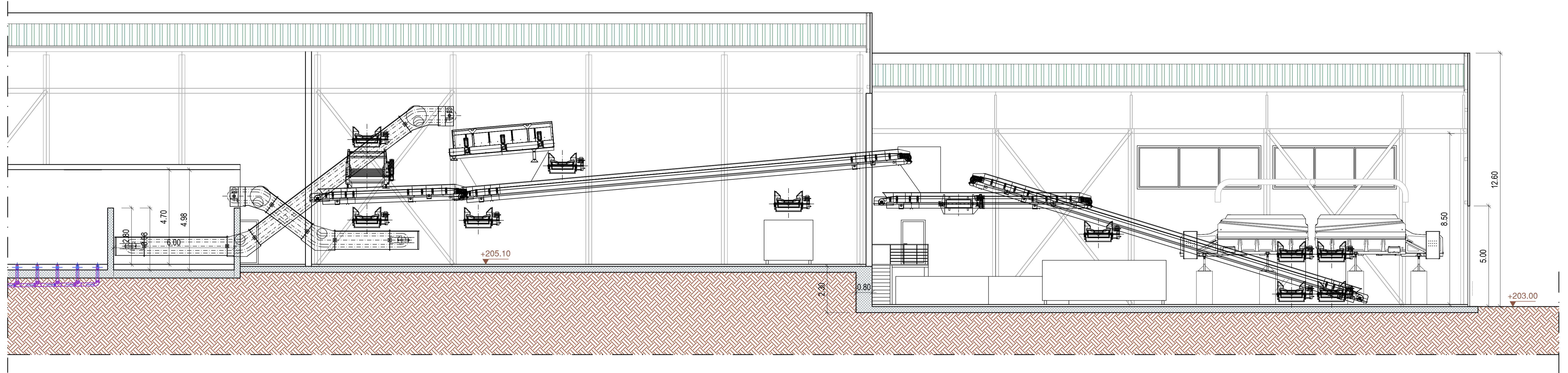
SEZIONE A-A
