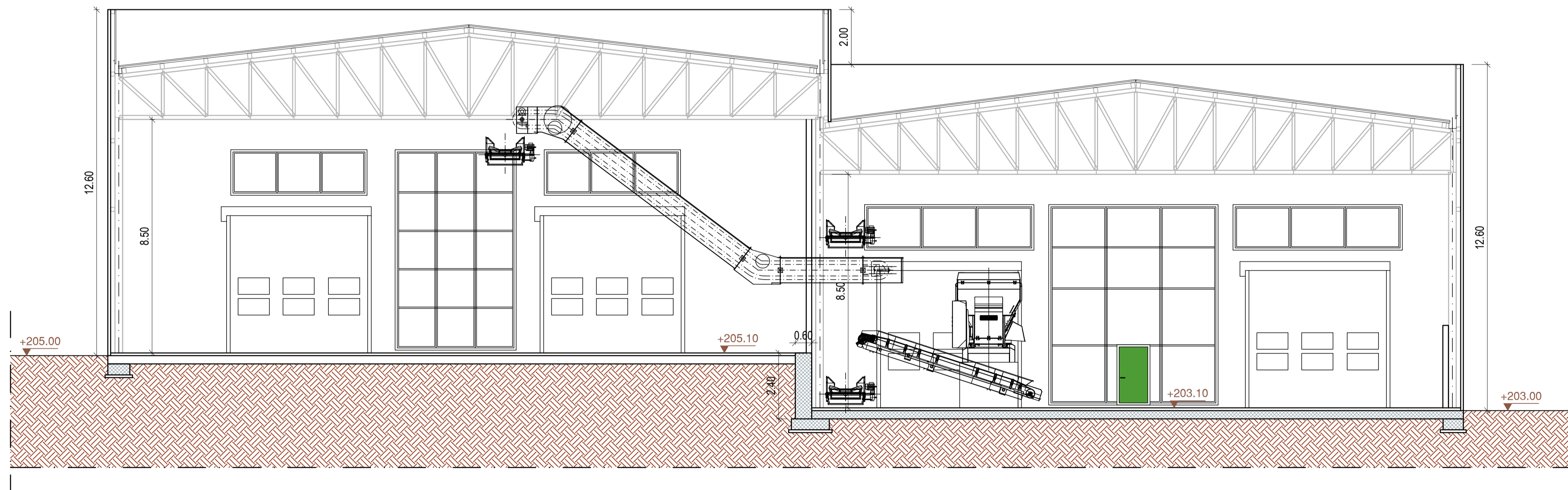
SEZIONE B-B
